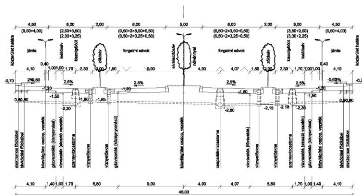
1. ábra B. III. a-A a-B B. IV. b-A Kösterületi tervek: belterületi főút M = 1 : 200 46 m szabályozási szélesség
