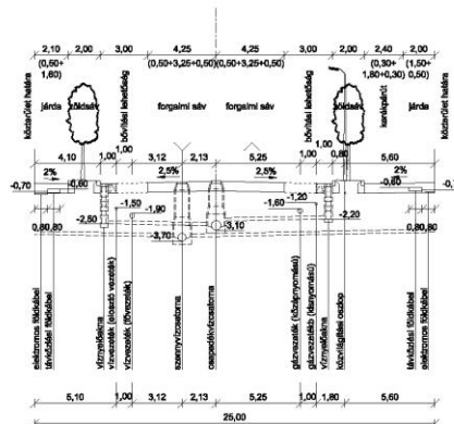
3. ábra B. III. a-C B. IV. b-B c-A Kösterületi tervek: belterületi főút M = 1 : 200 még elfogadható szabályozási szélesség: 25 m
